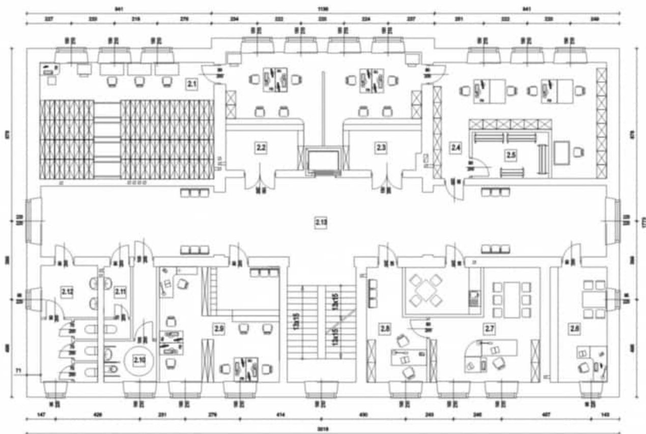
RZUT III PIĘTRA 1:100
